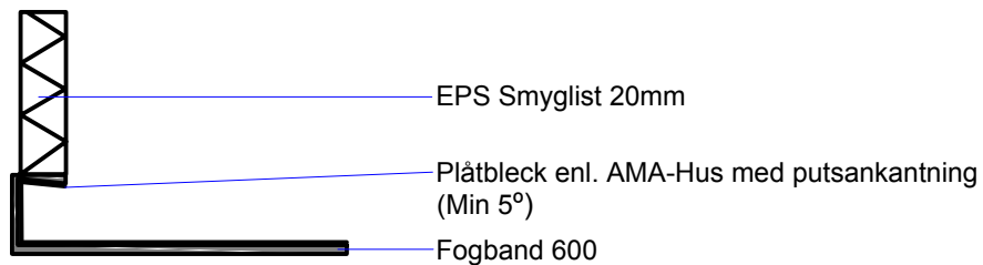
Frontvy Fönsterbleck
